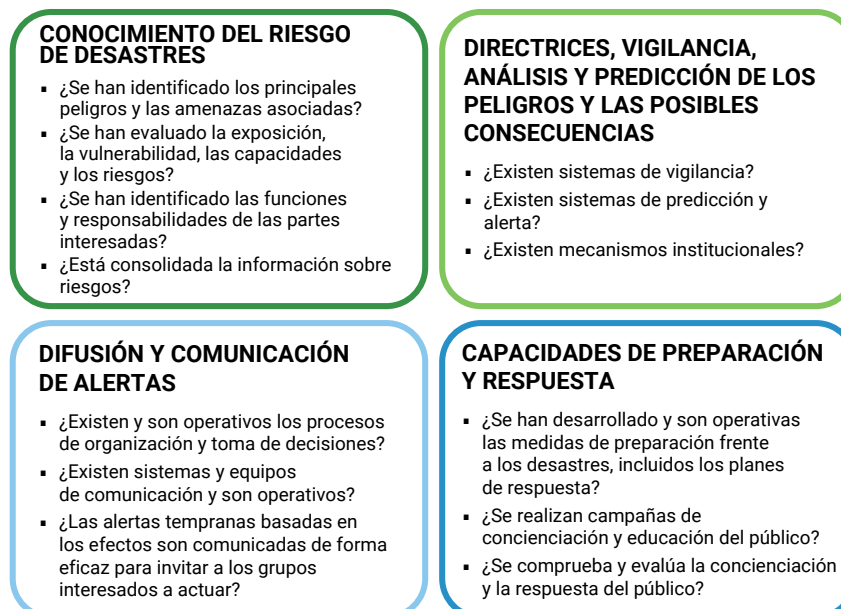
Figura 15. El concepto de la predicción centrada en las personas y basada en los efectos
