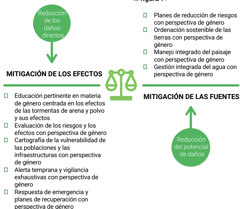
Figura 7. Un doble enfoque de la mitigación del riesgo de tormentas de arena y polvo para la reducción del riesgo de desastres
