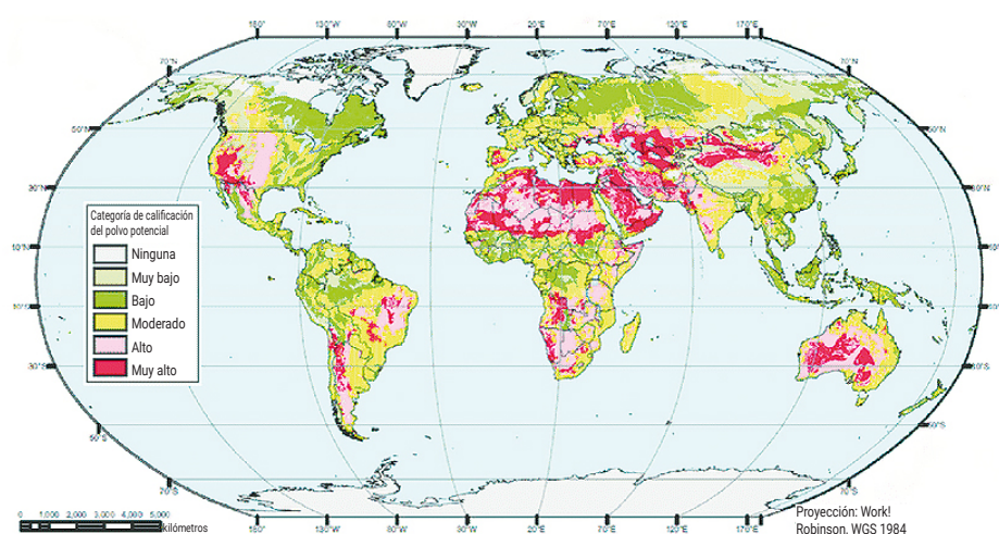
Figura 4. Zonas de emisión de tormentas de arena y polvo a nivel mundial
