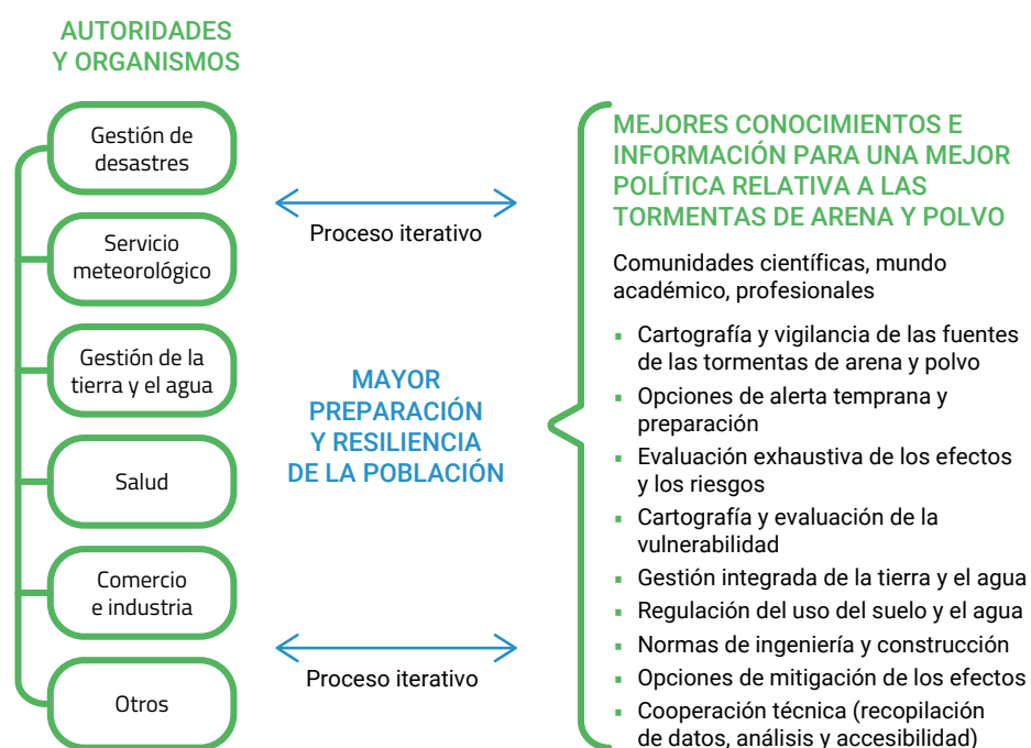
Figura 8. Marco de coordinación y cooperación para la gestión del riesgo de tormentas de arena y polvo
